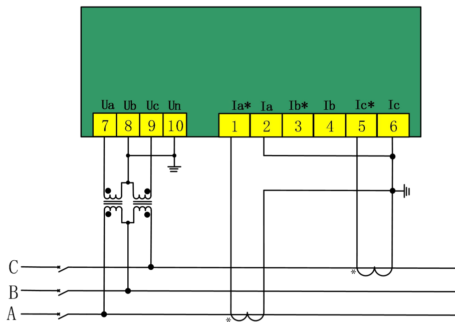
三相三线，2PT,2CT，B 相电流不显示
