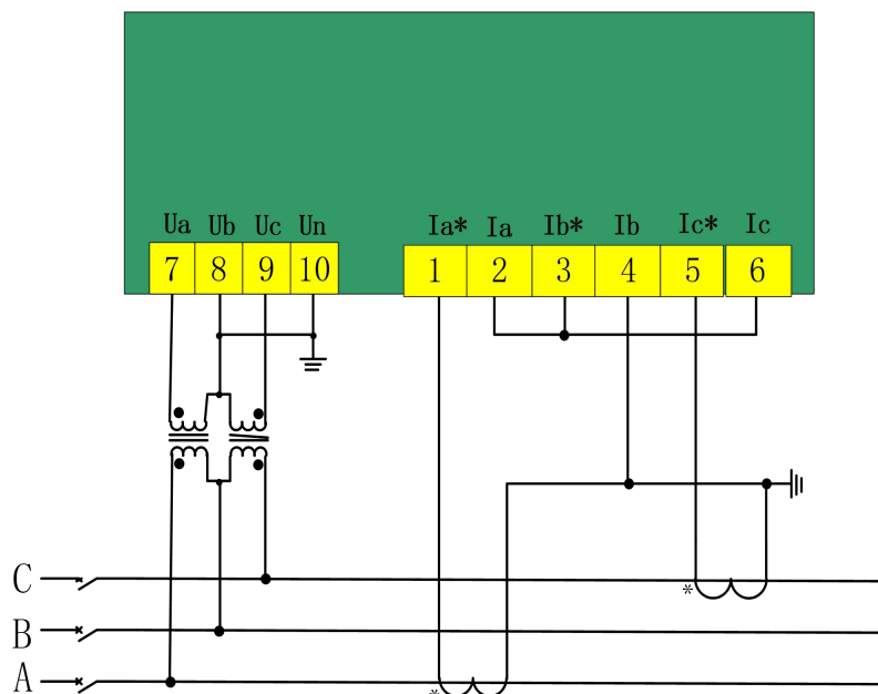
三相三线，2PT,2CT，B 相电流显示
