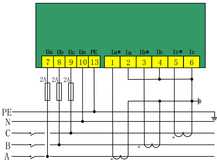
三相五线系统，无 PT,3CT
