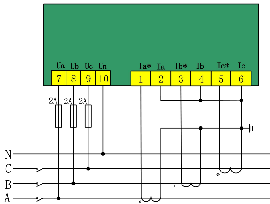
三相四线系统，无 PT,3CT
