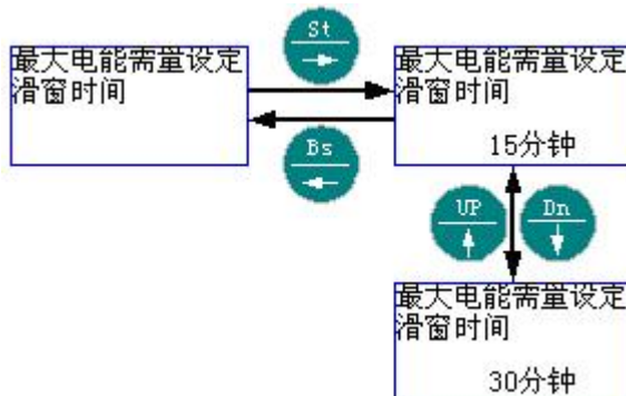
5.8.4 菜单结构 4: “最大电能需量设定” - “瞬时电能需量”
