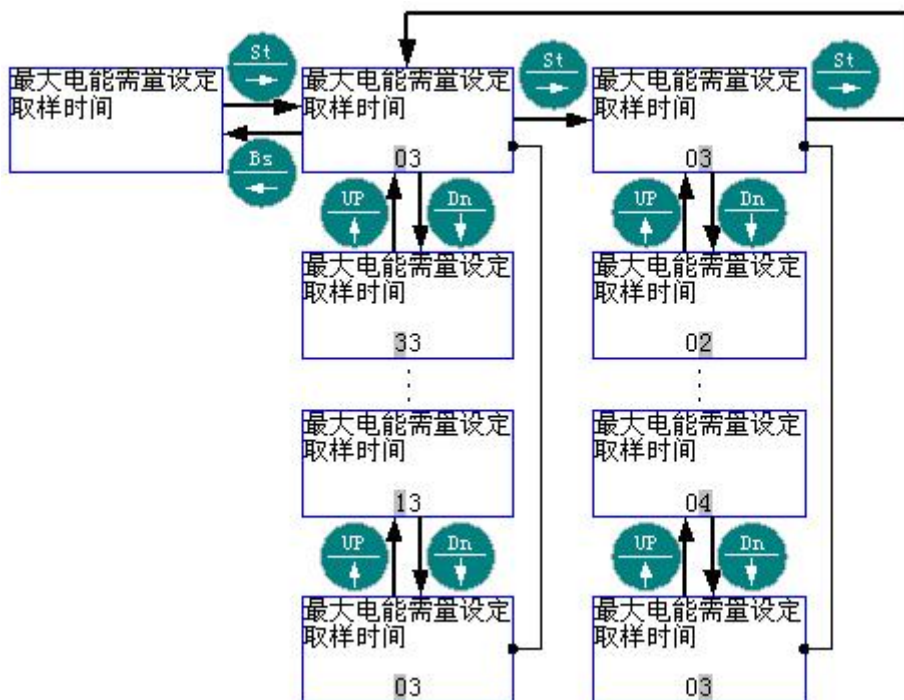
5.8.3 菜单结构 3: “最大电能需量设定” - “滑窗时间” (15 分钟、30 分钟)
