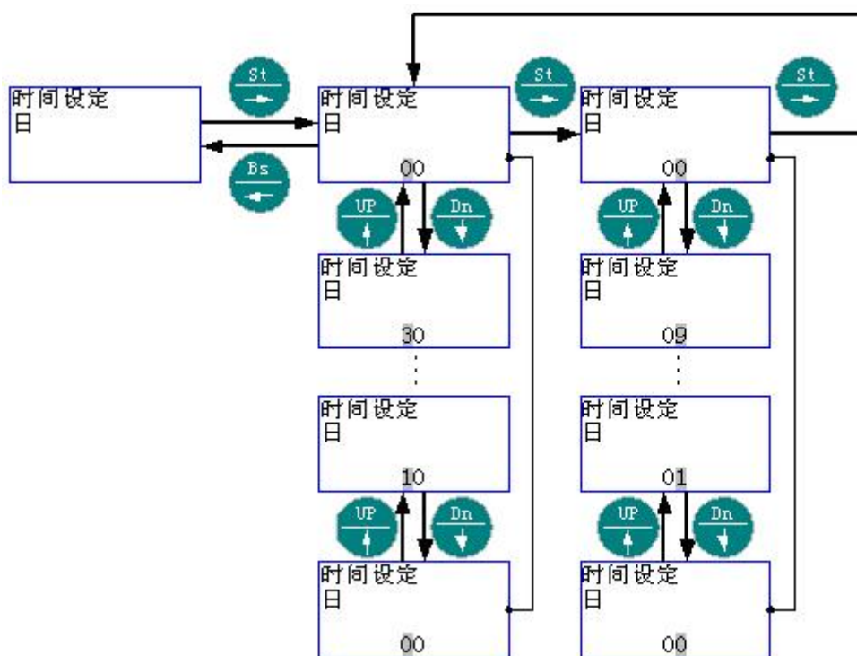
5.9.5 菜单结构 5: “时间设定” - “时”
