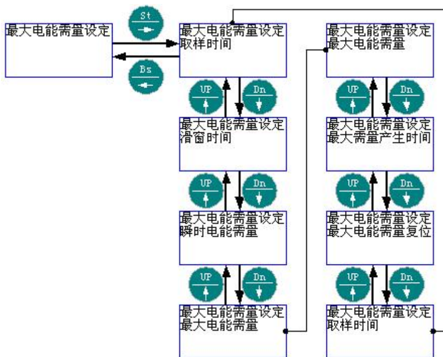
5.8.2 菜单结构 2: “最大电能需量设定” - “取样时间” (3~30 分钟)
