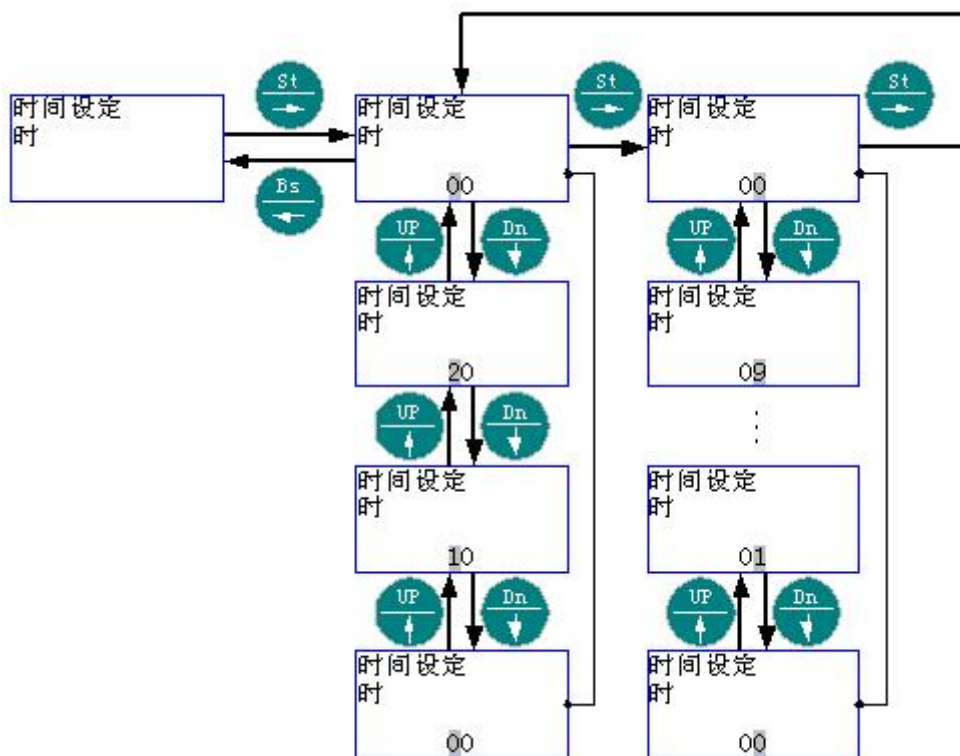
5.9.6 菜单结构 6: “时间设定” - “分”
