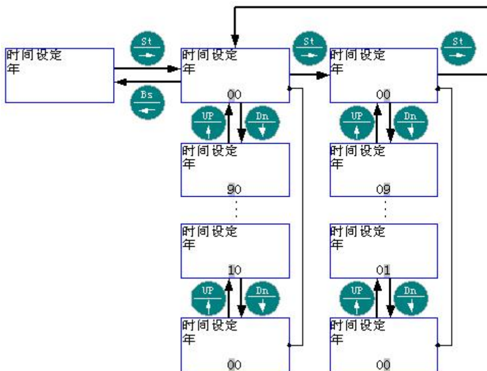
5.9.3 菜单结构 3：“时间设定” - “月”
